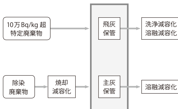
図2 焼却灰減容化フロー図
