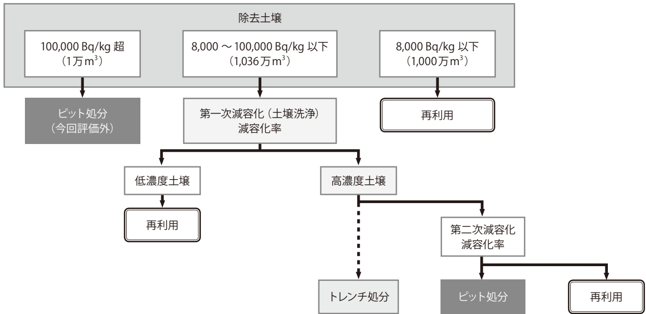
図 15 除去土壌の一次減容及び二次減容フロー
