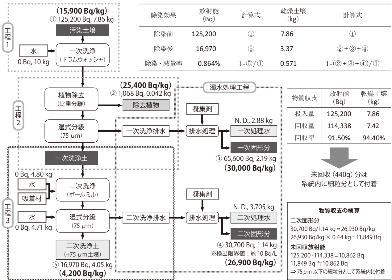
図 16 一次減容化技術の実証事業成果 (一例)
