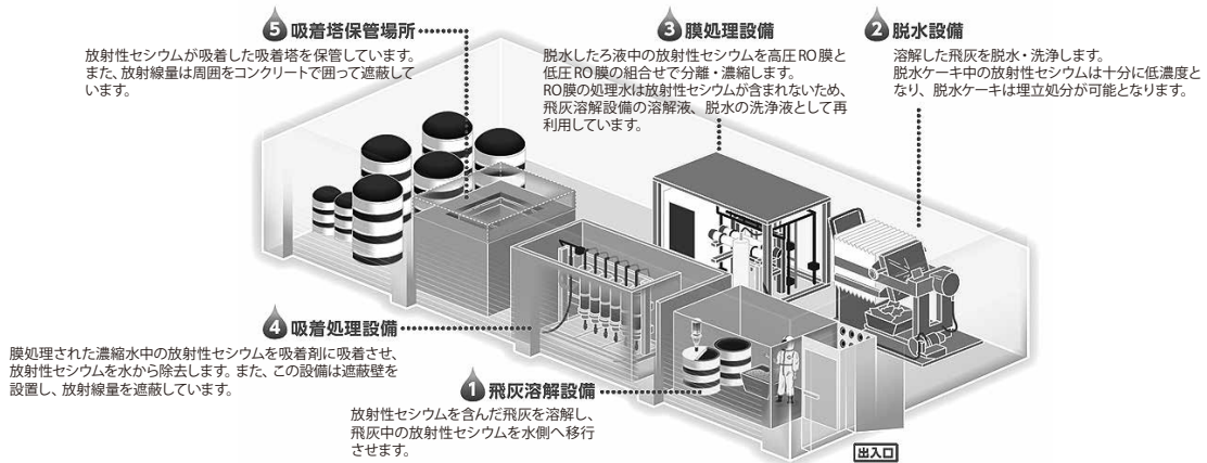
図3 焼却飛灰の減容化システム 国立研究開発法人 国立環境研究所/福岡大学/株式会社神鋼環境ソリューション
