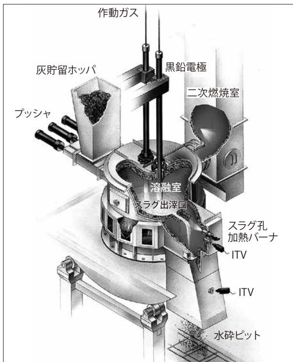
図4 焼却主灰の熔融減容化施設
