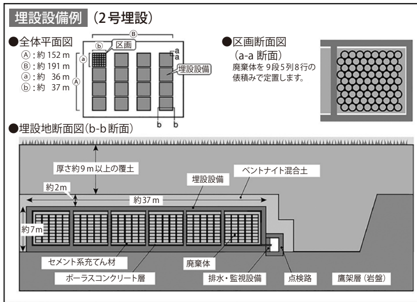
図8 ピット型処分構造図(日本原燃)
