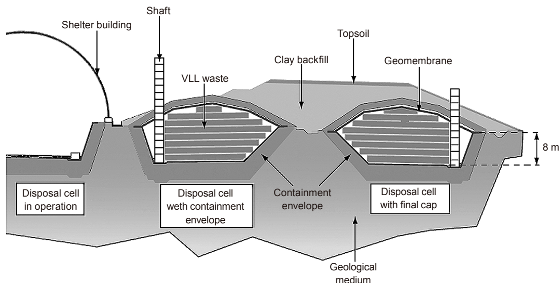
図7 トレンチ処分構造図(フランスのモルビリエ)
