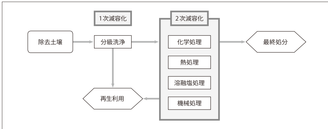
図5 除去土壌の減容化フロー図
