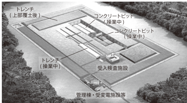
図12 研究施設等廃棄物の埋設処分場の完成予想図 出典: 国立研究開発法人 日本原子力研究開発機構のホームページ、「埋設事業の紹介」より転載 (URL: http://www.jaea.go.jp/04/maisetsu/aisatu/aisatu2.html )
